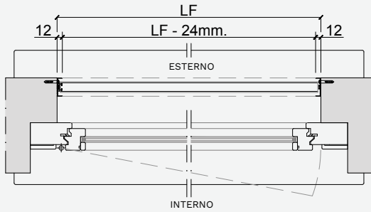
Carro chiuso con sistema ermetico
